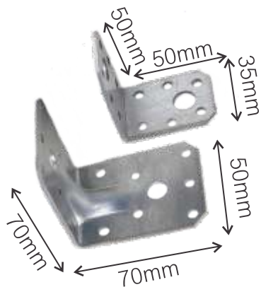
hoekplaat
