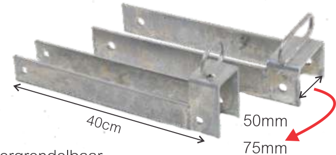
vergrendelbaar fermable
