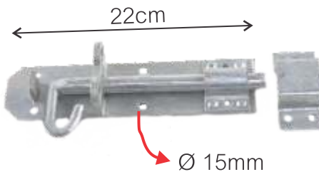
zware schuifgrendel gegalvaniseerd verrou lourd galvanisé
