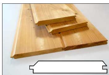
TWTG17142 Thermo rain/languette 17 x 142 mm largeur utile : 130 mm
