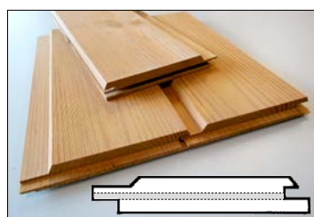
TWPL19140 Thermowood planchette raboté, rainuré aux 4 bouts 19 x 140 mm largeur utile : 130 mm
