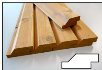
TWSR2668 Thermosiding bardage 26 x 68 mm, raboté lisse, largeur utile : 55 mm
