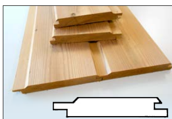
TWTG19140 Thermo rain/languette 19 x 140 mm fixation invisible !, largeur utile : 130 mm
