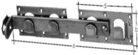
Verrou double bichromaté
