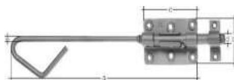
Verrou à queue zingué 32cm
