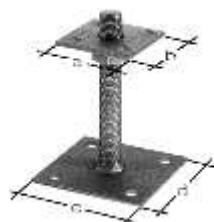
Support bichromaté à cheviller réglable en hauteur de 30 à 150mm
