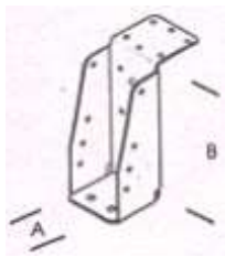
Connecteurs de poutre zingués 50x125mm 63x175mm 75x225mm
