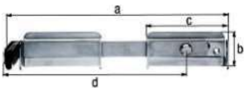
Verrou double inox
