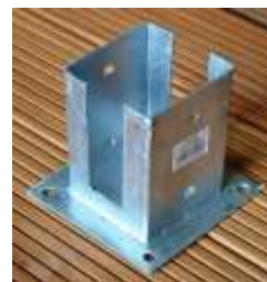
Ancre sur platine galvanisée à cheviller avec fentes pour poteaux rainurés
