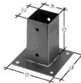
Ancre sur platine galvanisée à cheviller 71mm 91mm 121mm
