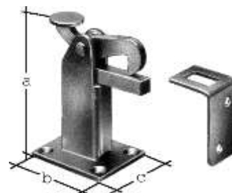
Verrou « IDEAL » bichromaté
